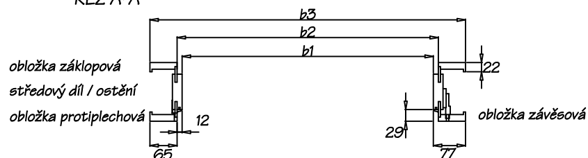
ŘEZ A-A
