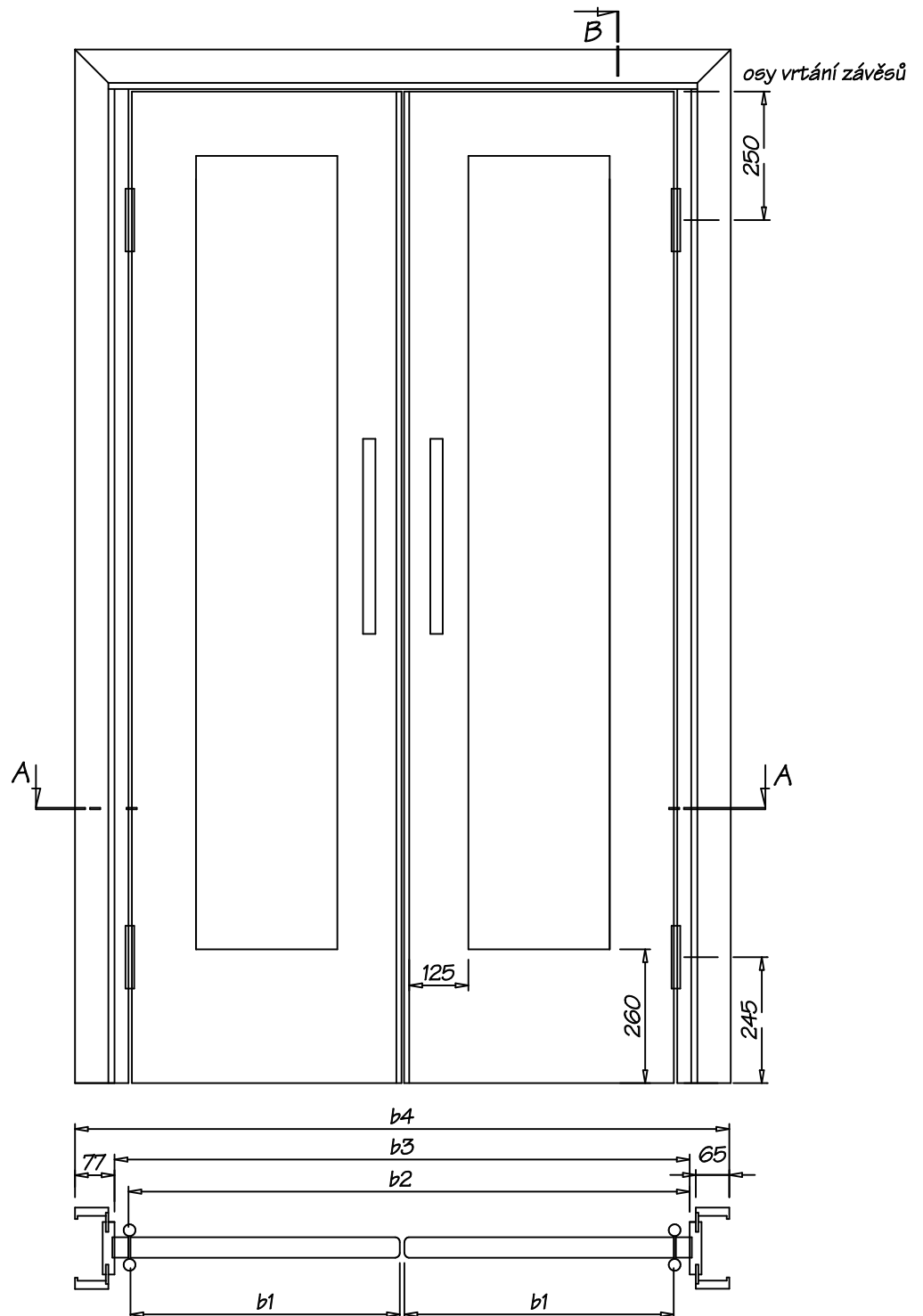
ŘEZ A-A
